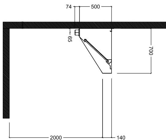
Boční
